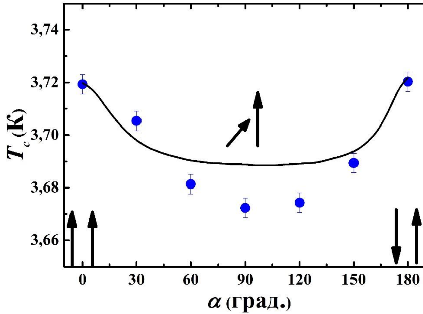
Рис. 3. Образец \text{CoO}_x/\text{Py1}(3 \text{ нм})/\text{Cu}(4 \text{ нм})/\text{Py2}(1.7 \text{ нм})/\text{Cu}(2 \text{ нм})/\text{Pb}(70 \text{ нм}) с нулевым стандартным эффектом спинового клапана ( \Delta T_c^{\text{P}} = \Delta T_c ). Угловая зависимость T_c(\alpha) , вызванная дальнедействующей триплетной компонентой сверхпроводящего конденсата, показана кружками. Сплошная линия – теоретическая кривая.
