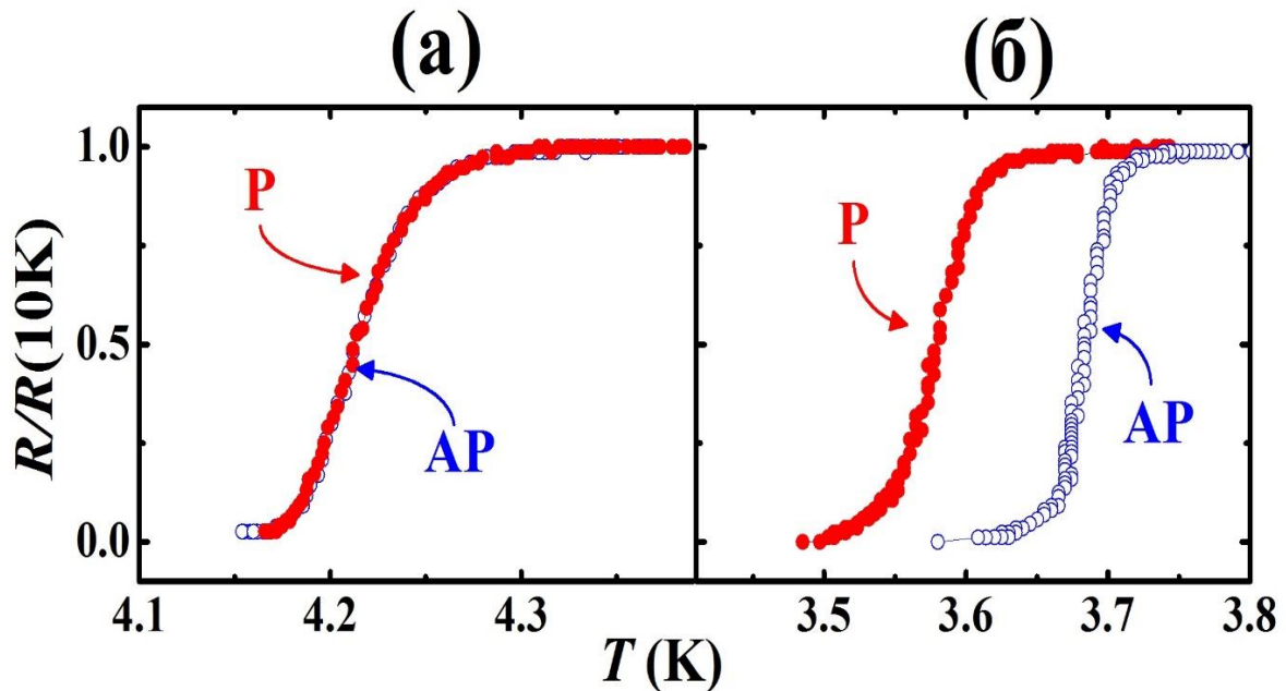
Рис. 1. Сверхпроводящие переходы, измеренные при AP ( \circ ) и P ( \bullet ) ориентациях намагниченностей ферромагнитных слоев, для образцов \text{CoO}_x/\text{Py}1(3 \text{ нм})/\text{Cu}(4 \text{ нм})/\text{Py}2(1 \text{ нм})/\text{Cu}(2 \text{ нм})/\text{Pb}(70 \text{ нм}) с шероховатым (а) и гладким (б) сверхпроводящим слоем
