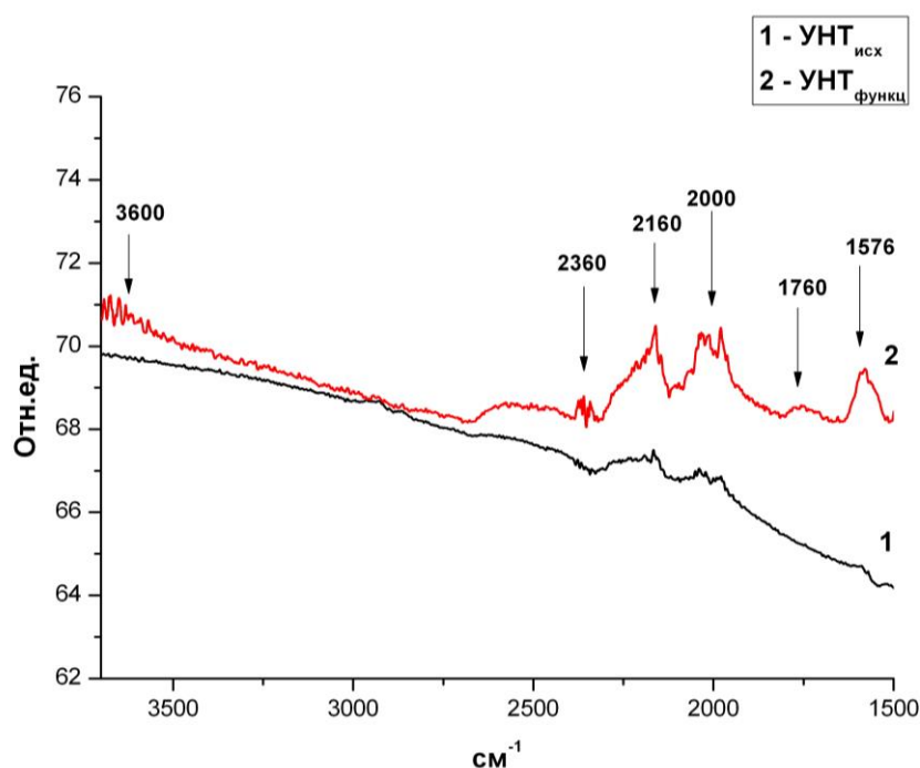
Рис.2 – ИК-спектры исходных (1) и функционализированных (2) углеродных нанотрубок.
