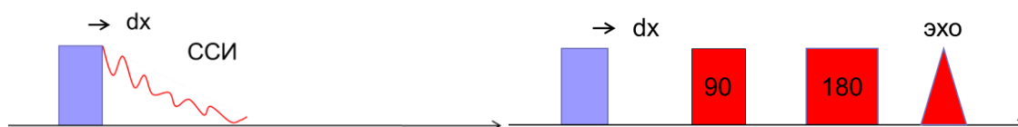
Рис.1 Импульсные последовательности
