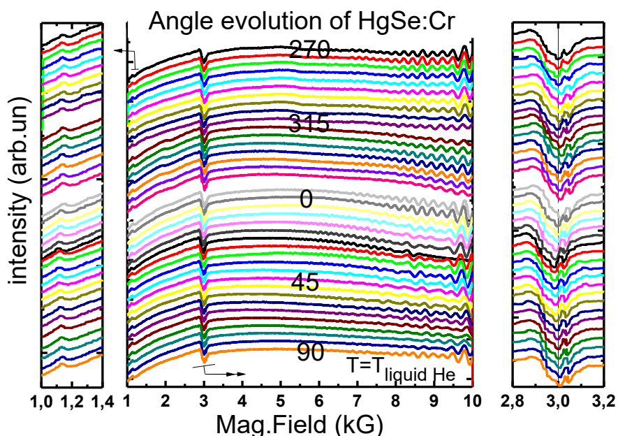
Рис.2 Угловая эволюция интенсивности магнитной восприимч. HgSe:Cr.
