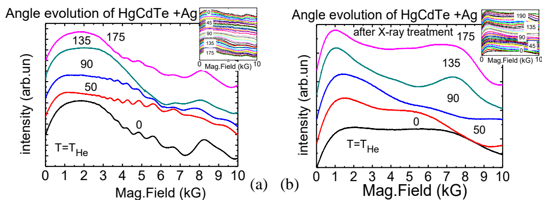
Рис.2 Угловая эволюция интенсивности магнитной восприимчивости HgTeCd:Ag в произвольной ориентации кристалла (a) после X-ray облучения, вращение в магнитном поле перпендикулярном оси вращения C_4 (b).
