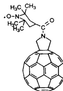
Рис.3 Структура фуллерен-радикал
