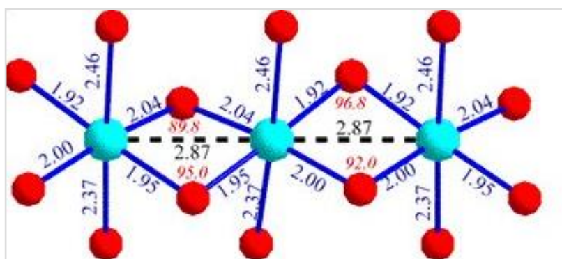
Рис. 1 Модель \text{CuO}_6 цепочки в \text{LiCuSbO}_4 [6]
