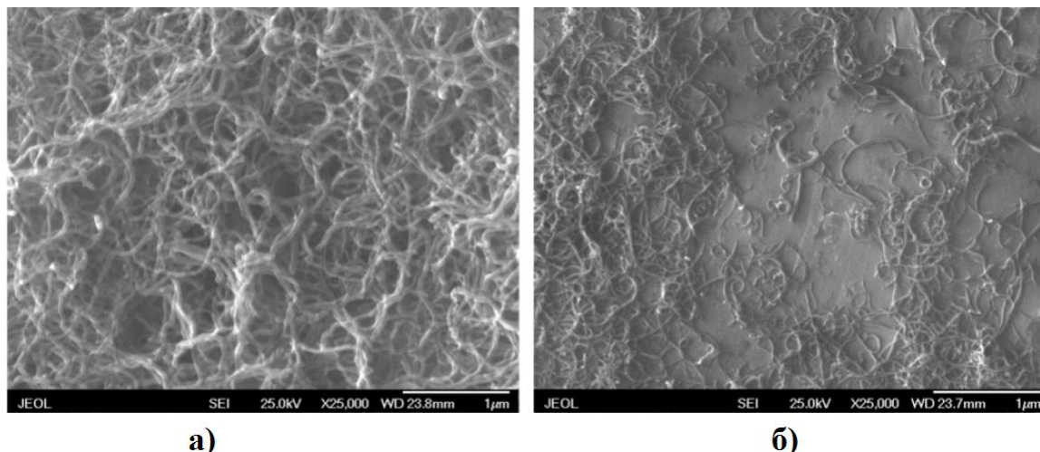
а) б) Рис. 1 – Электронные микрофотографии исходных (а) и модифицированных (б) углеродных нанотрубок.
