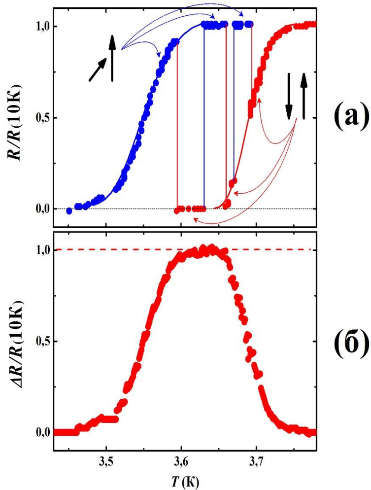
Рис. 2. (а) Переключение между нормальным и сверхпроводящим состояниями для образца \text{CoO}_x/\text{Py}1(3 \text{ нм})/\text{Cu}(4 \text{ нм})/\text{Py}2(1 \text{ нм})/\text{Cu}(2 \text{ нм})/\text{Pb}(70 \text{ нм}) путем медленного понижения температуры в пределах \Delta T_c и резкого изменения направления магнитного поля \alpha между 180^\circ (красные кружки) и 90^\circ (синие кружки). (б) Температурная зависимость \Delta R = R(\alpha = 90^\circ) - R(\alpha = 180^\circ) , демонстрирующая полное переключение сверхпроводящего тока в температурном интервале 3.6 – 3.66 К
